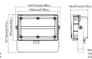
15W&27W(Trunion Mount)
