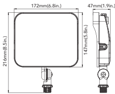
15W&27W(Knuckle Mount)
